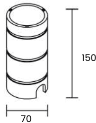
Code : JC990 Outer-case for: CALLA, LILIUM, DATURA, MINI GLICINE, GLICINE, JUNCUS
