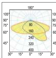
ASY 1 Asimetrico - Asymmetric
