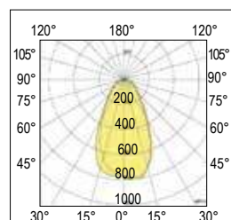
90° Diffondente - Flood
