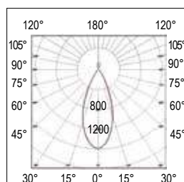
40° Diffondente Diffusing
