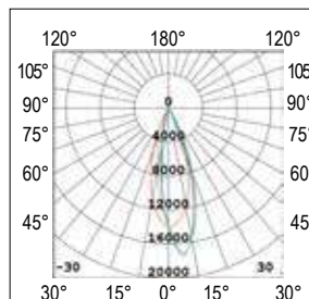
25° Concentrante - Spot
