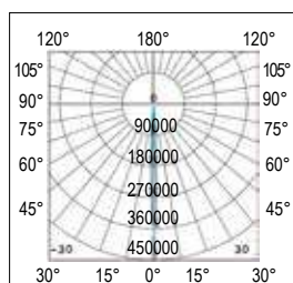
4° Concentrante Narrow
