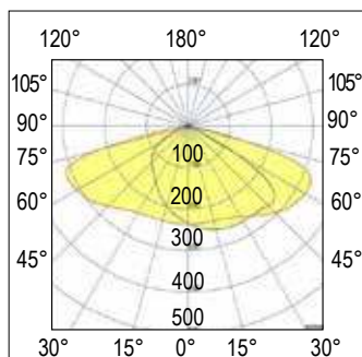
ST/CDL4 Ottica consigliata per illumi- nazione stradale Optic recommended for street lighting
