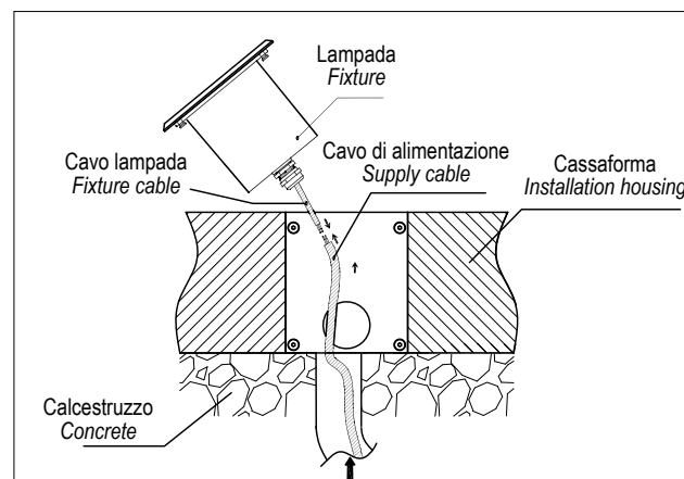
Versione con ottica diffusore completo di vetro antiscivolo Diffuser optics versions complete with non-slip glass
