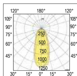
40° Semi-diffondente - Wide
