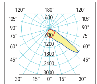
ASY Asimmetrico - Asymmetric
