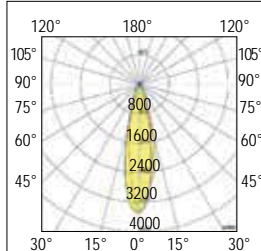
25° Concentrante - Spot
