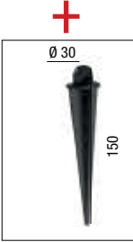
Cod. 24165 Picchetto in alluminio Aluminum picket
