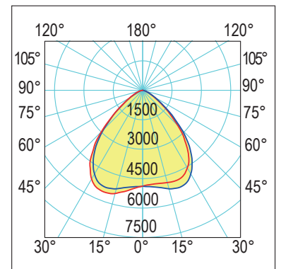
90° Diffidente - Wide
