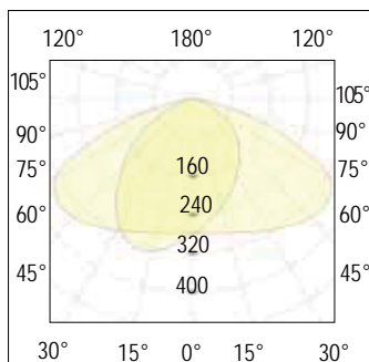
Ottica di serie Standard optic
