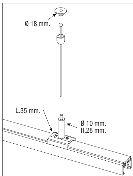
Kit sospensione con staffa corta e tenditore automatico, cavo 3m in acciaio Ø 1,5 mm. Suspension kit with short bracket and automatic gripper, 3m cable in steel Ø 1.5 mm.
