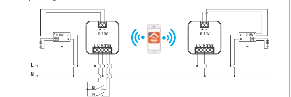
Anschlussplan - Diagramme de connexion
