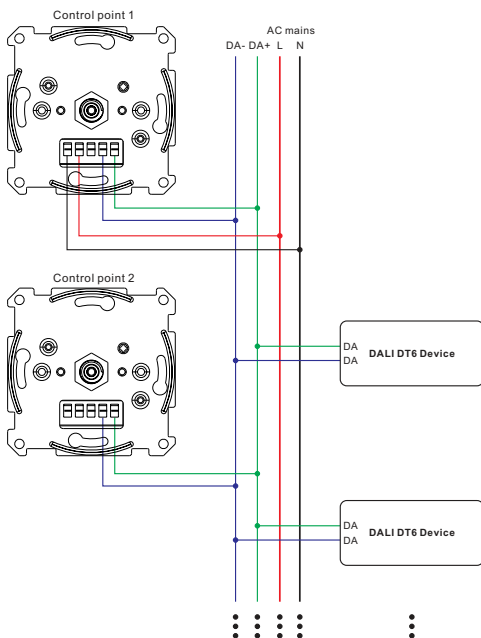
Schema di collegamento - Wiring diagram
