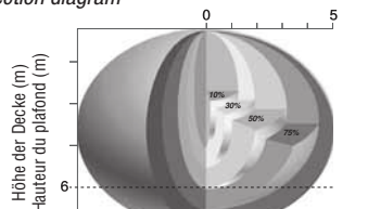
Erfassungsschema für die Deckenmontage (m) Schéma de détection plafond (m)
