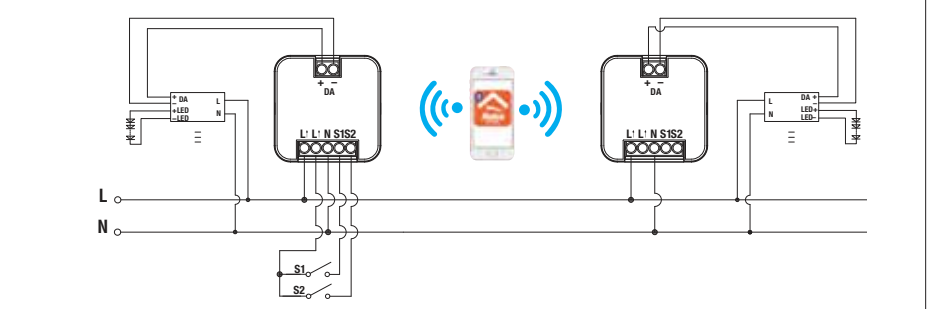
Schema di collegamento - Wiring diagram
