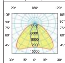
Ottica Ellittica Elliptical optics
