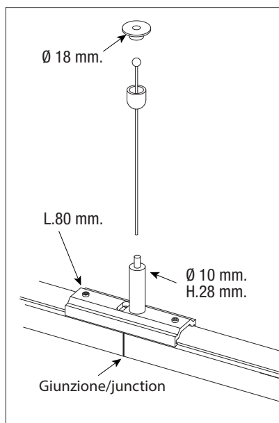
Kit sospensione con staffa lunga e tenditore automatico per giunzione fila continua, cavo 3m in acciaio Ø 1,5 mm. Suspension kit with long bracket and automatic gripper for continuous row junction, 3m cable in steel Ø 1.5 mm.
