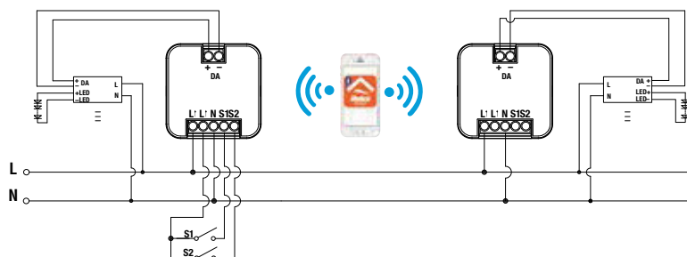
Schema di collegamento - Wiring diagram
