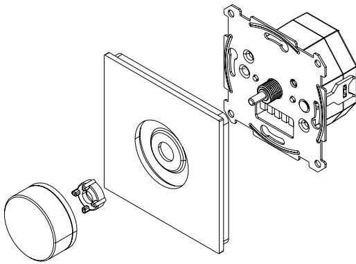
Schema di collegamento - Wiring diagram
