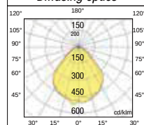
Ottica diffondente Diffusing optics
