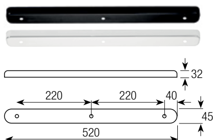
ROSONE RETTANGOLARE 3 FORI RECTANGULAR CEILING ROSE - 3 HOLES
