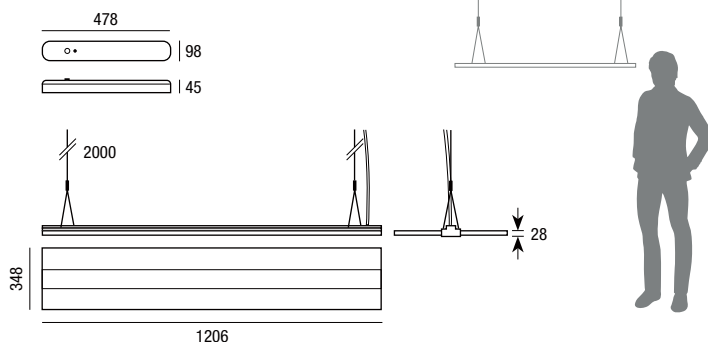
Selettore 2CCT interno al rosone. 2CCT selector inside the ceiling rose.
