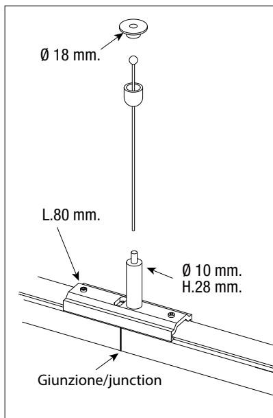
Kit sospensione con staffa lunga e tenditore automatico per giunzione fila continua, cavo 3m in acciaio Ø 1,5 mm. Suspension kit with long bracket and auto- matic gripper for continuous row junction, 3m cable in steel Ø 1.5 mm.
