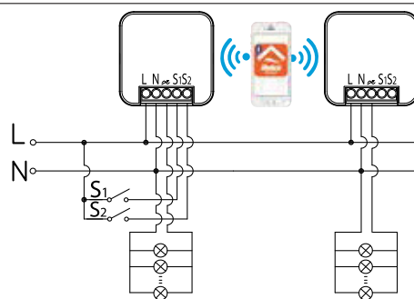
Schema di collegamento - Wiring diagram
