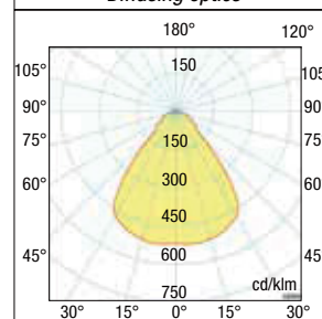
Ottica diffusa Diffusing optics
